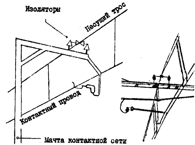
С х е м а 38. Контактная сеть железной дороги
