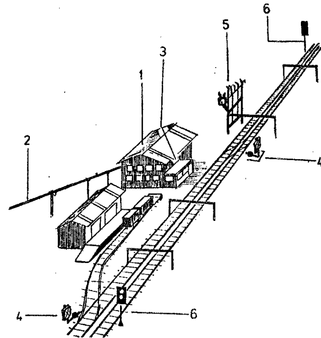
С х е м а 45. Оборудование железнодорожной станции: 1 - здание станции; 2 - линия телефонной связи; 3 - диспетчерская; 4 - переводные стрелки; 5 - главная опора контактной сети с масляным изолятором; 6 - семафоры
