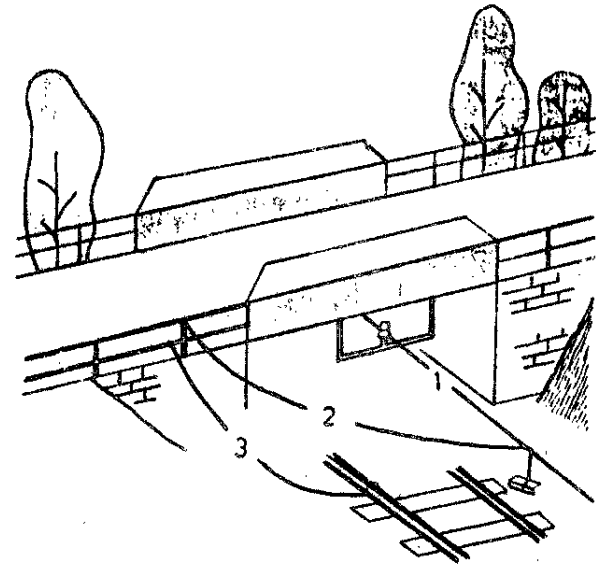
С х е м а 39. Устройство короткого замыкания на контактной сети:
