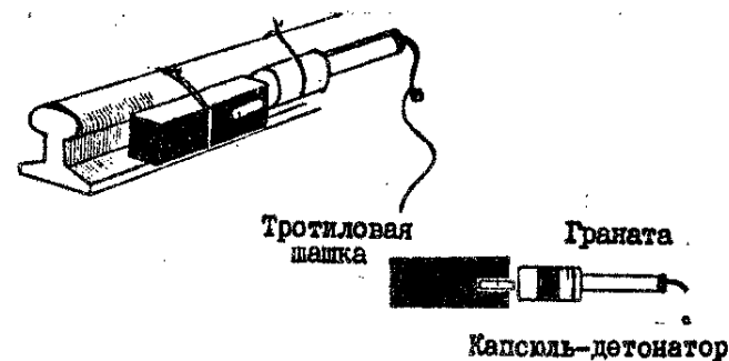
С х е м а 41. Подрыв рельса:
